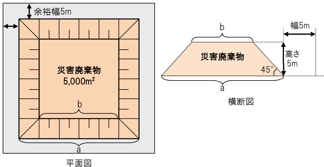
【図2-9】 仮置場面積の模式図
