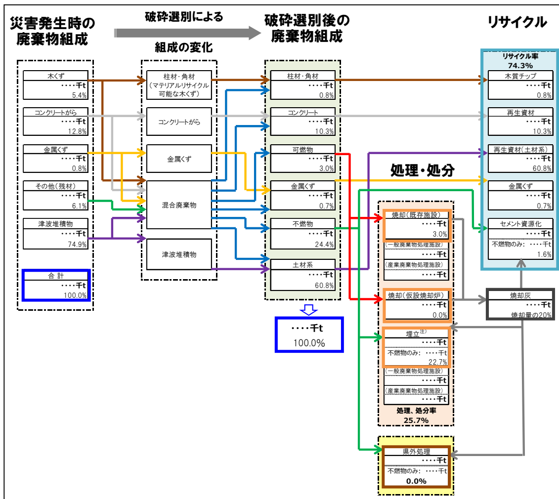
【図2-8】 沖縄県南東沖地震3連動の災害廃棄物処理フロー（例）
