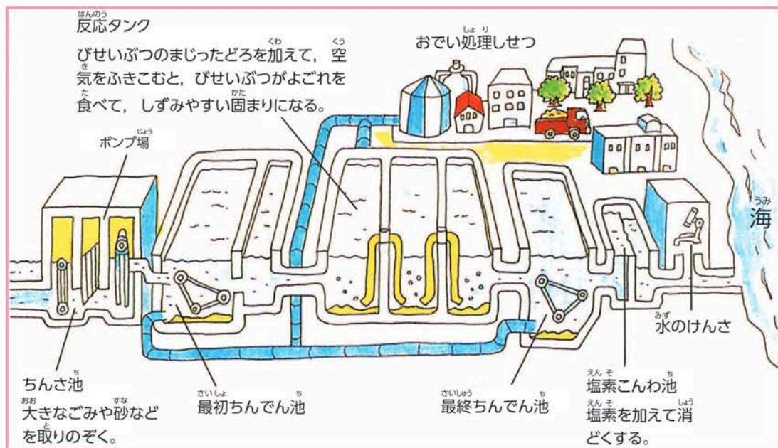
下水処理しせつのしくみ
