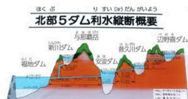
↑ 地下でつながる5つのダム
