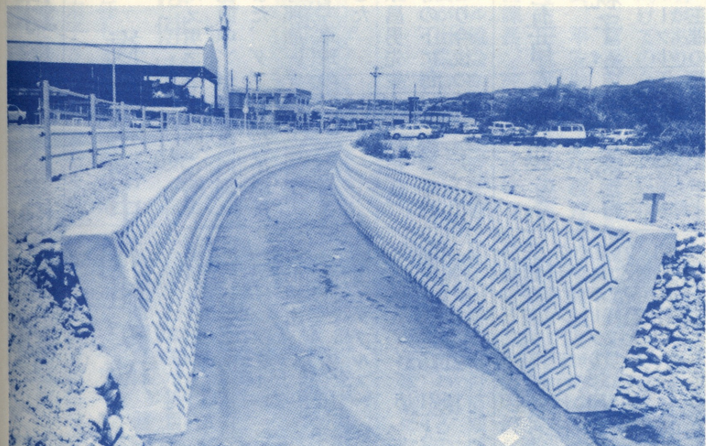
稲国川排水路整備工事 工事費5,030万円、延長340.7m、幅員1.2m～4.6m、深さ1.1m～2.0m、写真は3工区＝工業専用地域内
