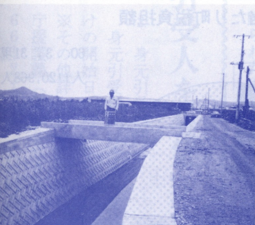
池田地区農地保全整備事業 総事業費一億一五〇万円、排 水路九一五メートル、水兼農道五三 五メートル、ガードレール七〇メートル、 ガードフェンス一〇九メートル整備
