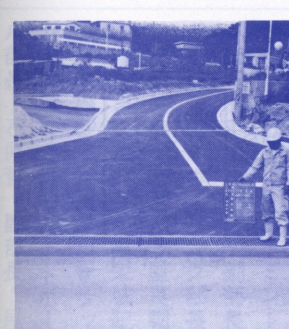
上原線道路改良事業 総事業 費八〇二万円、延長四〇〇 メートル、幅員七・五
