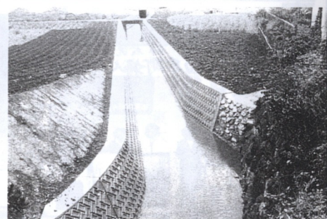
幸地川災害復旧工事(徳佐田地内) 工事費2560万円、延長131.6メートル、幅員5.1メートル、高さ2.6メートル
