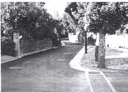
嘉手苅地内部落道整備工事 工事費900万円、延長256メートル、幅員4メートル
