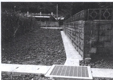
津花波地内排水路整備工事 工事費1,200万円、延長336メートル、W600×H600
