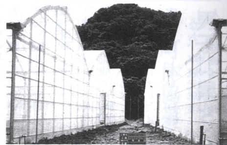
新農業構造改善事業(共同利用温室工事) 工事費3163万円、面積4068平方メートル(ハウス6棟)
