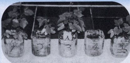
各ポイントの植物発育状況 毎年、死魚がでるポイント4では芽がでない
